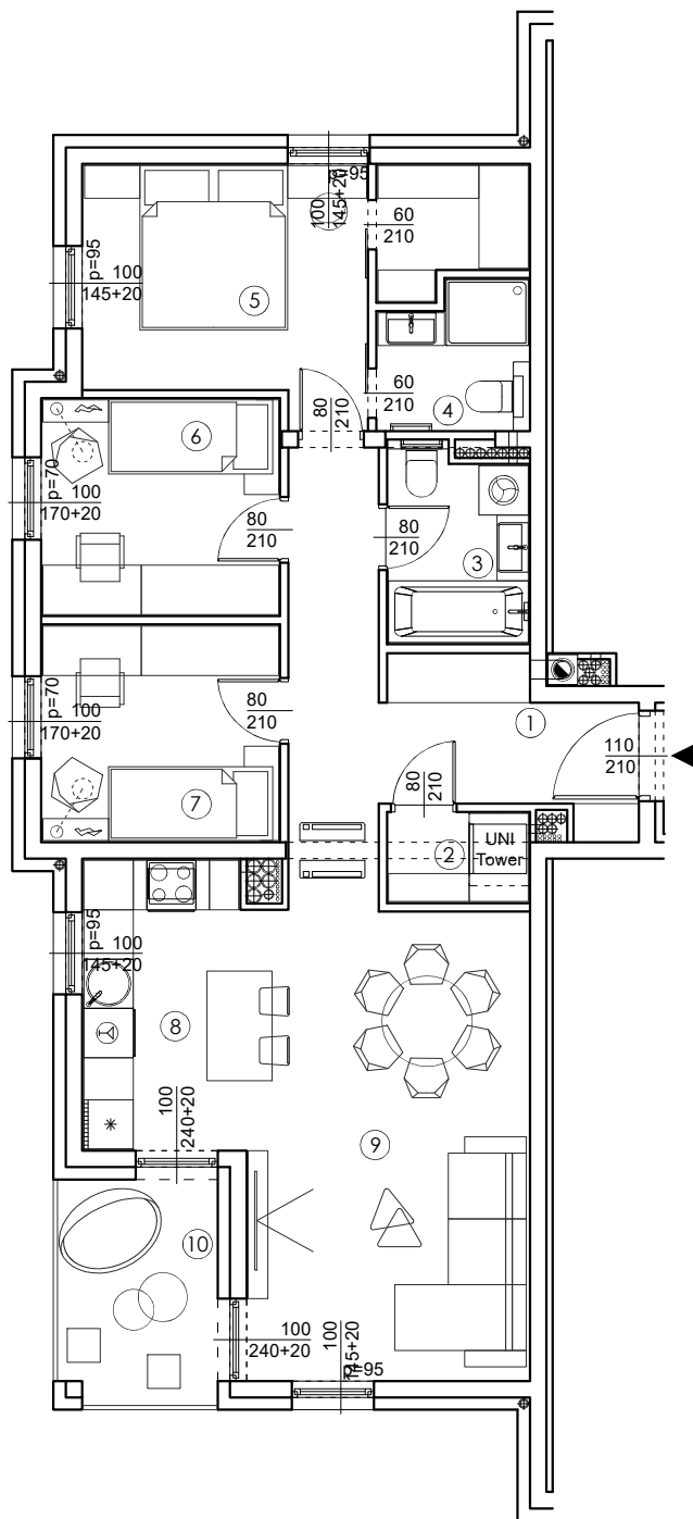
T 4-11 | 4-sobni stan
